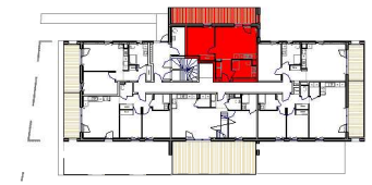
PLAN DU NIVEAU RDC
